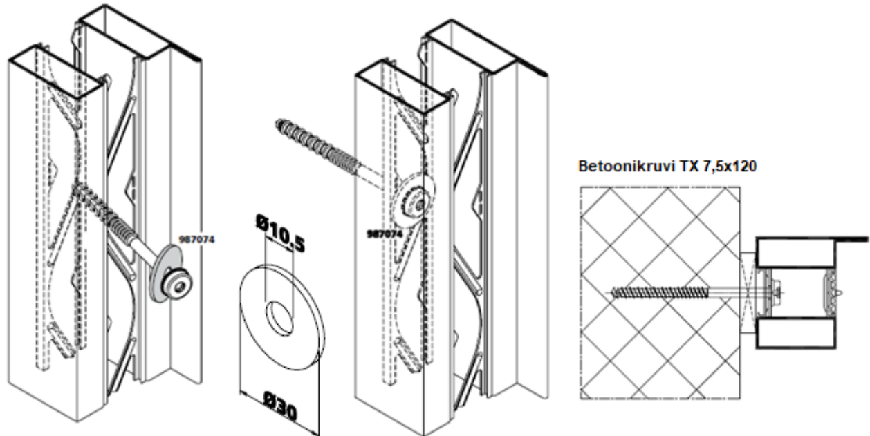
SKEEM 2 K-3 (Forsteri) kinnitamine paigaldusel.
